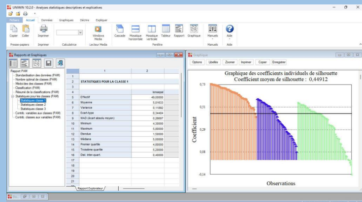
Graphique K-médoïdes
